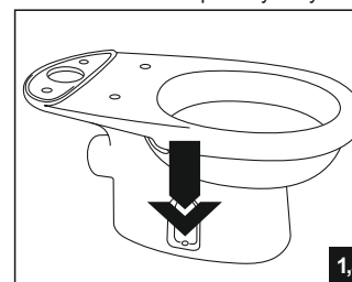
1,а Закрепить унитаз, используя комплект крепления, согласно схеме монтажа находящейся в комплекте крепления;
