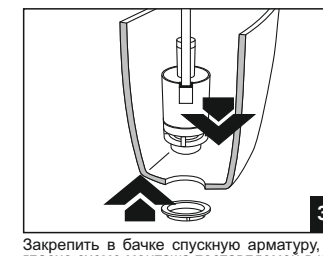
3,а Закрепить в бачке спускную арматуру, согласно схеме монтажа поставляемой в комплекте арматуры, подключить унитаз-комплект к канализации и системе холодного водоснабжения;
