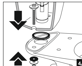
4,а Надеть прокладку. Установить бачок на унитаз и прикрепить его с помощью болтов;
