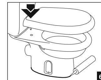
6,а Закрепить на унитаз сиденье согласно схеме сборки (поставляется в комплекте с сиденьем). При необходимости нанести герметик в зазор между полом и унитазом.
