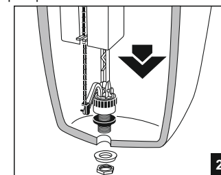
2,а Установить в бачке наполнительную арматуру, согласно схеме монтажа поставляемой в комплекте арматуры;
